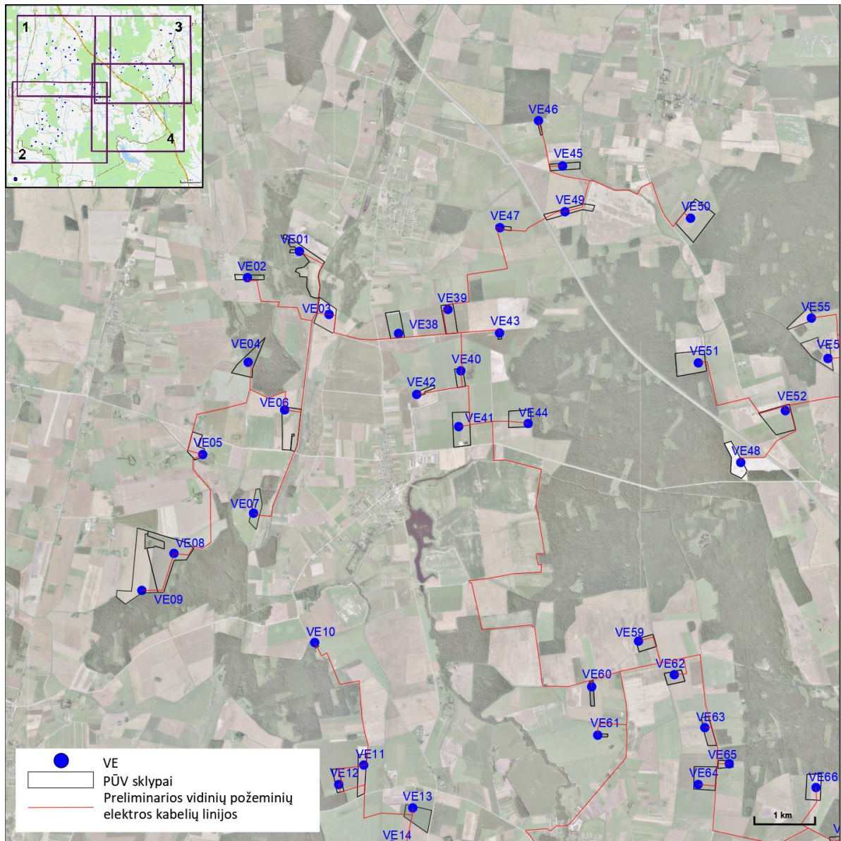
1 pav. Planuojamos preliminarios vidinių požeminio elektros kabelių linijos
