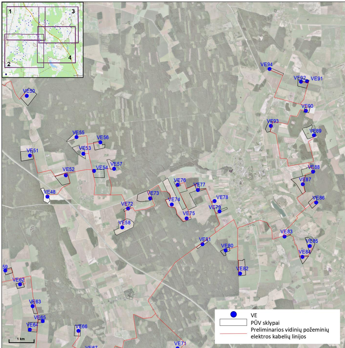
3 pav. Planuojamos preliminarios vidinių požeminio elektros kabelių linijos
