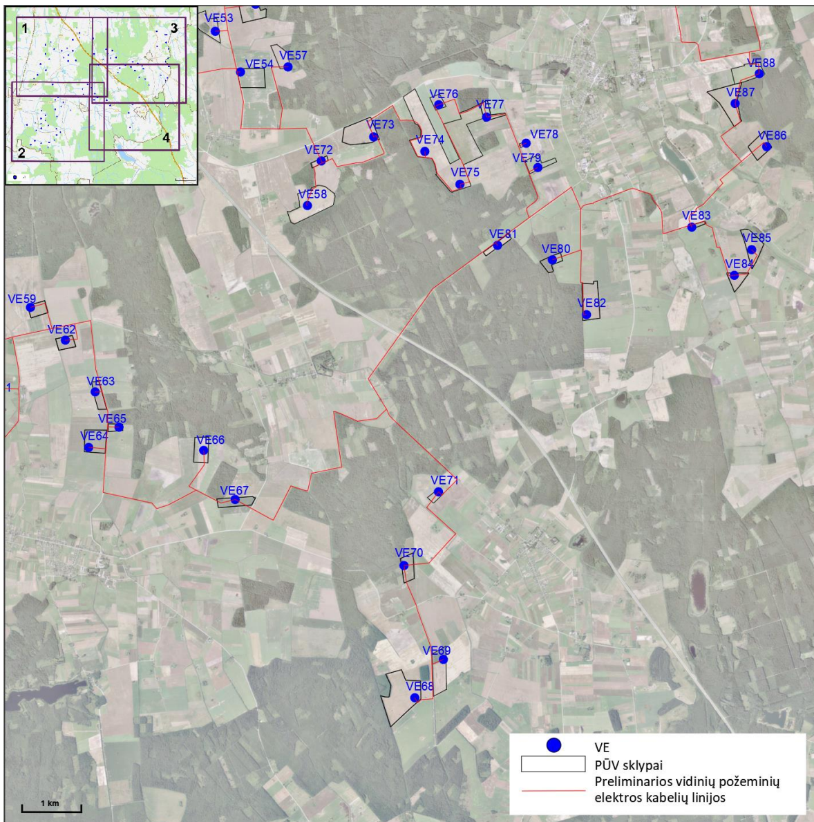
4 pav. Planuojamos preliminarios vidinių požeminio elektros kabelių linijos
