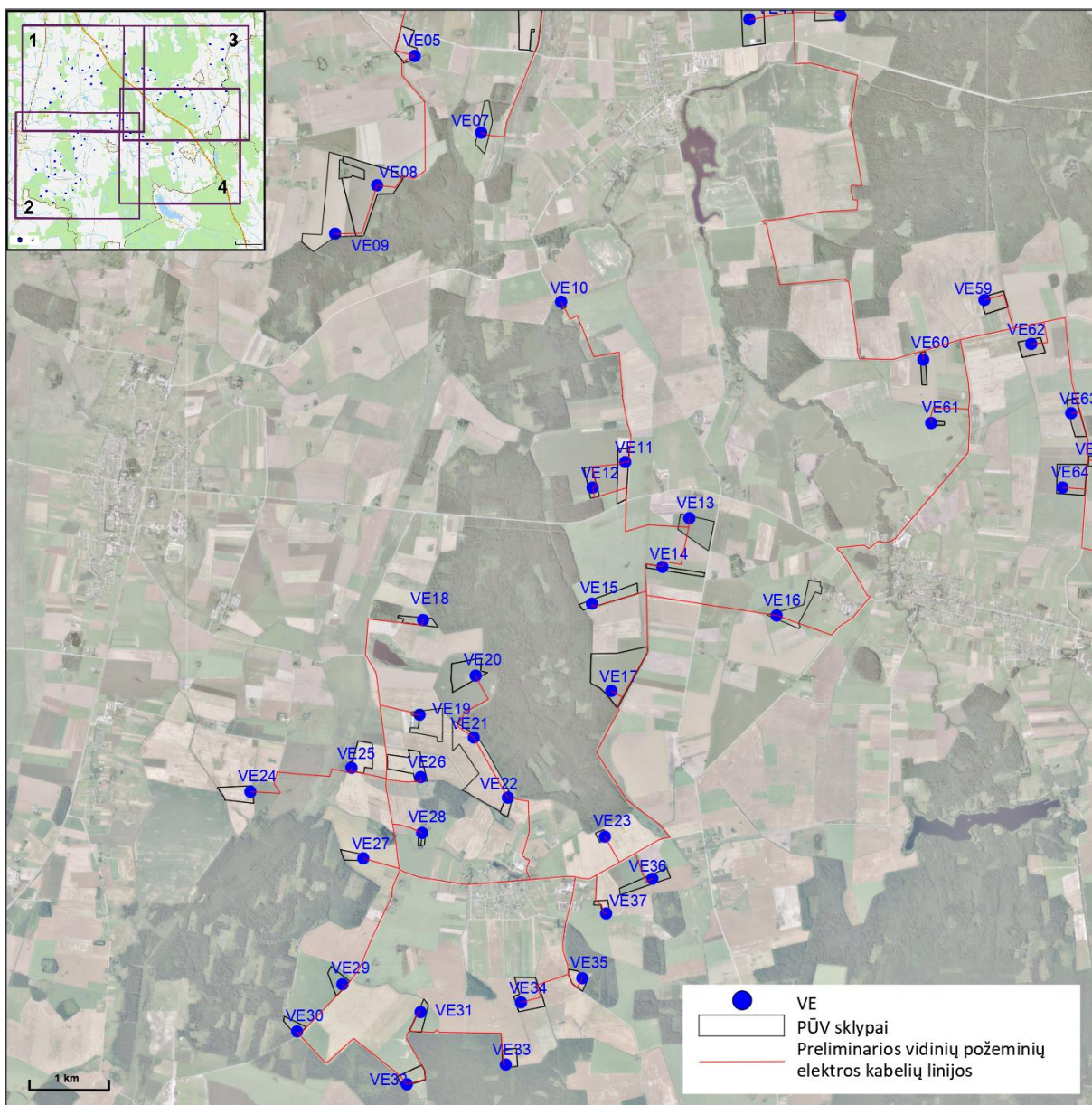
2 pav. Planuojamos preliminarios vidinių požeminių elektros kabelių linijos
