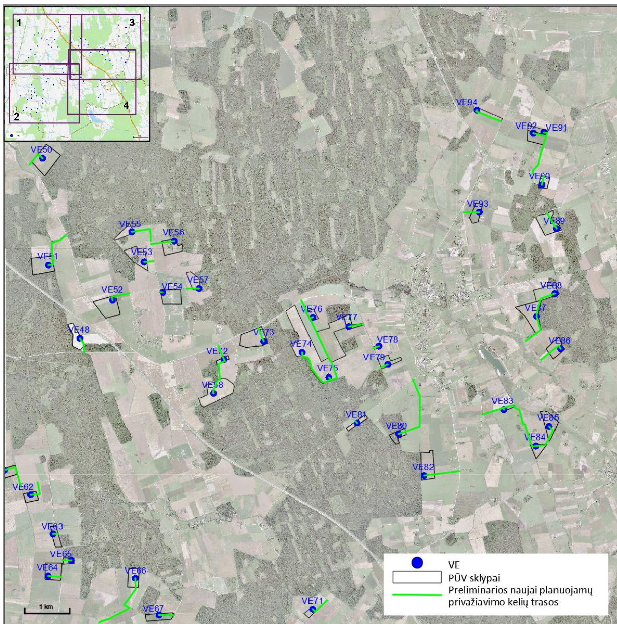
3 pav. Preliminarios naujai planuojamų privažiavimo kelių trasos
