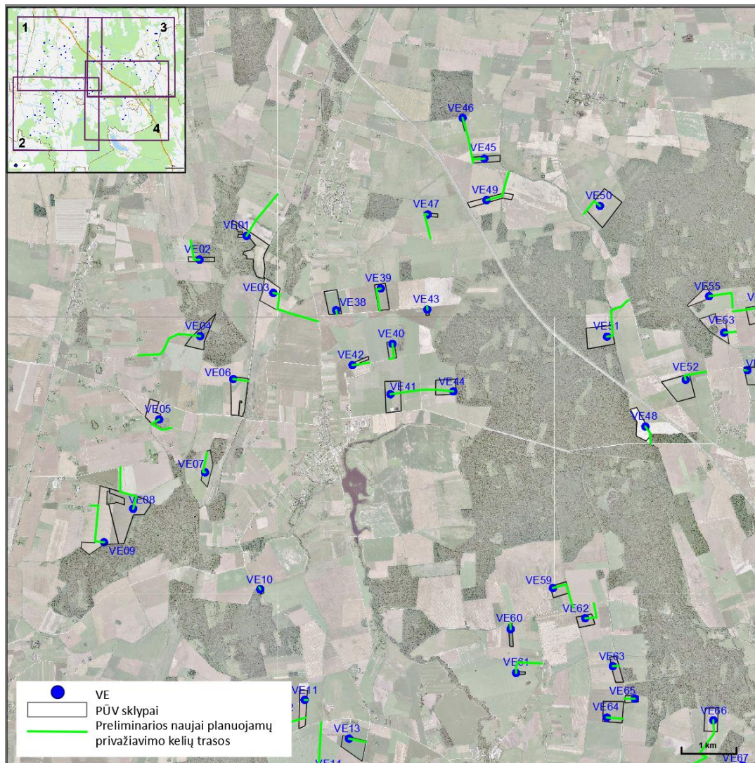
1 pav. Preliminarios naujai planuojamų privažiavimo kelių trasos
